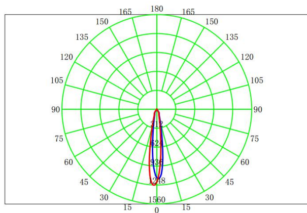
配光曲线
