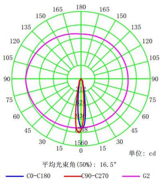
配光曲线
