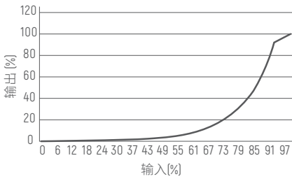
调光曲线
