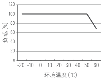
降额曲线
