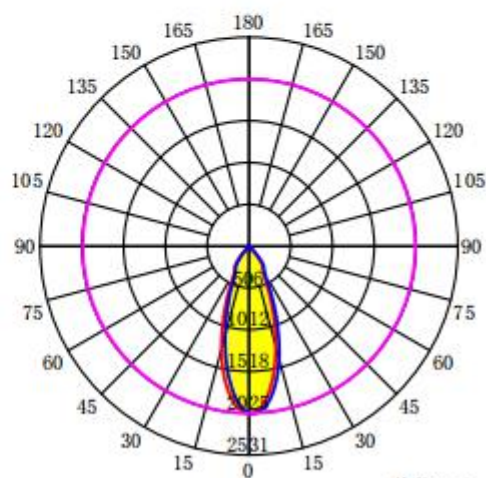
配光曲线
