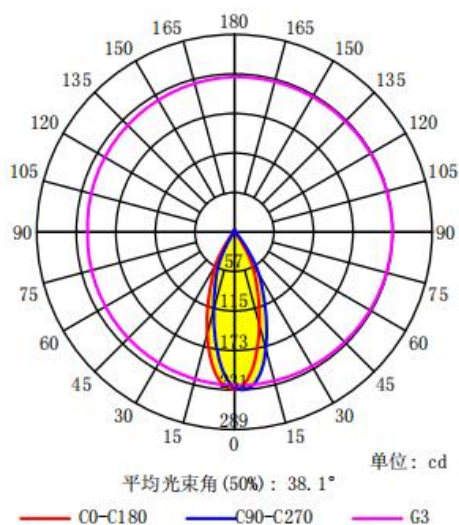
配光曲线
