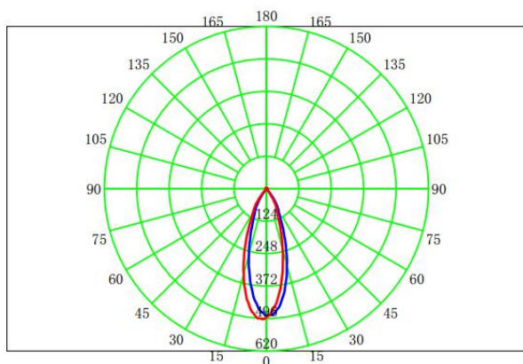
配光曲线
