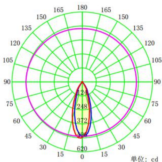
配光曲线
